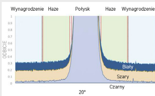
Informacje goniofotometryczne profilujące odbicie od białych, szarych i czarnych paneli z identyczną powłoką nawierzchniową.
