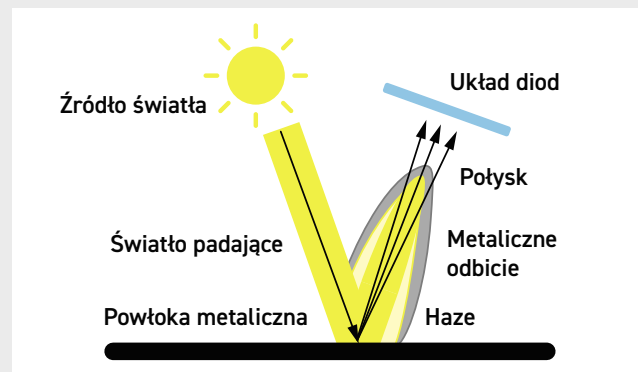
Wersja Novo-Gloss 20/60/85 z zamgleniem przechwytuje informacje kompensacyjne z obszaru przylegającego do kąta pomiaru zamglenia. Oznacza to, że może być stosowany na powłokach metalicznych, które odbijają światło.
